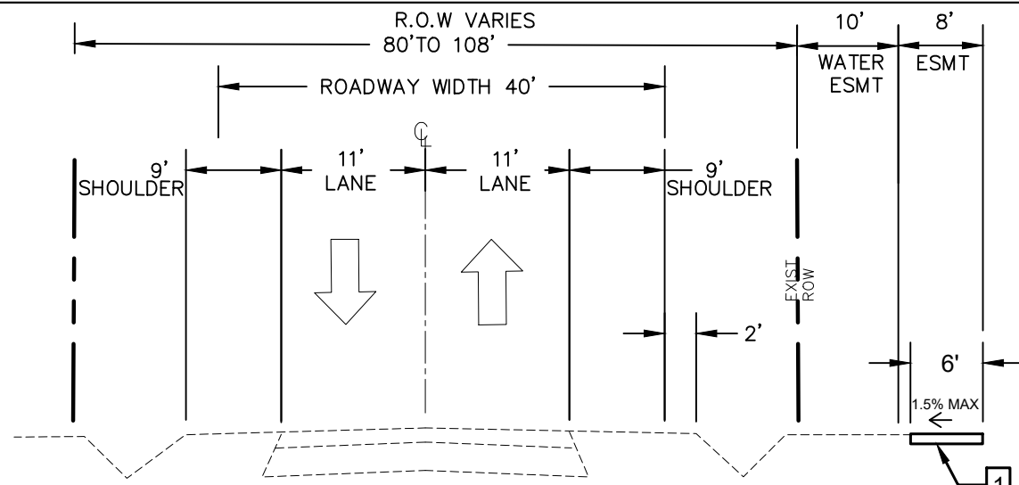
FM 1409 - PROP TYPICAL SECTION STA 61+00 TO STA 64+00
