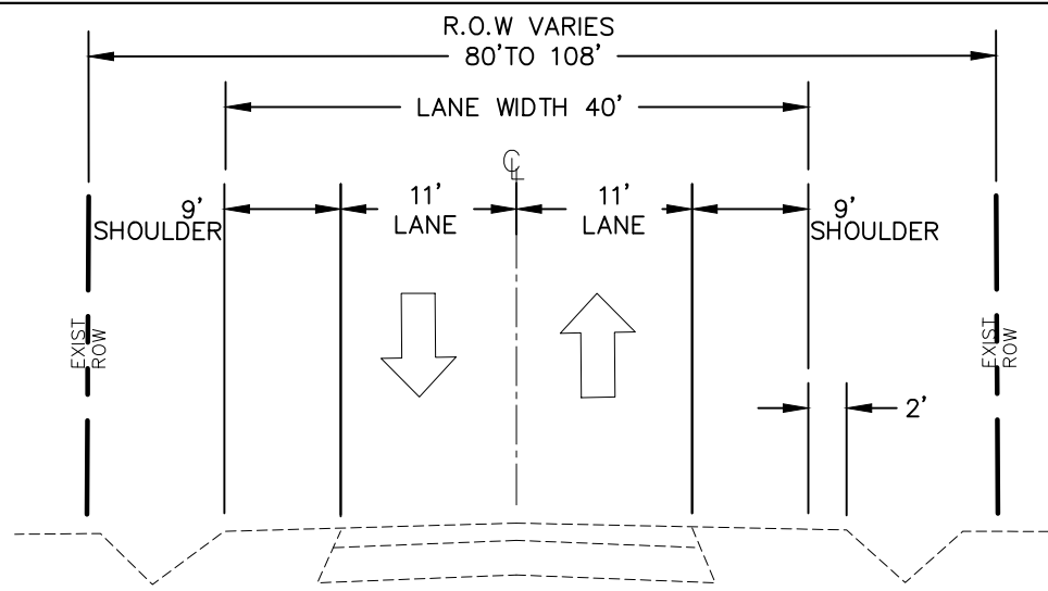
FM 1409 - EXIST TYPICAL SECTION STA 61+00 TO STA 64+00
