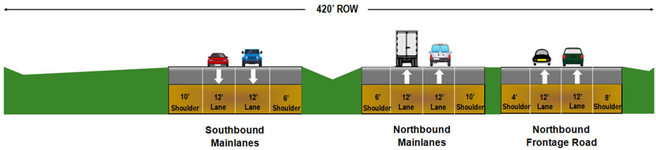
Sección Típica Existente
